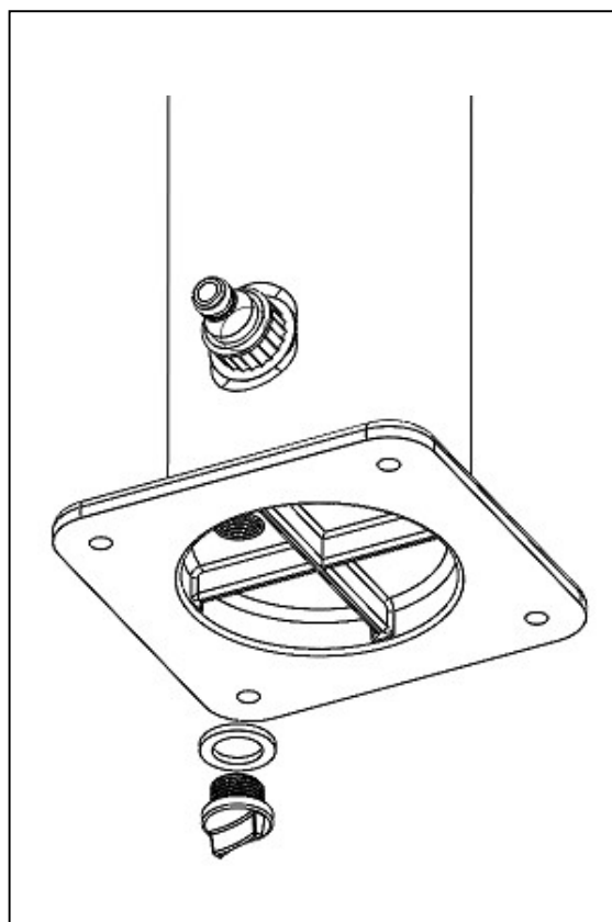
Obrázek 2 – Vypouštěcí zátka
